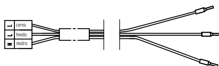
17. Kabel X2 (sestava) - 3414347
